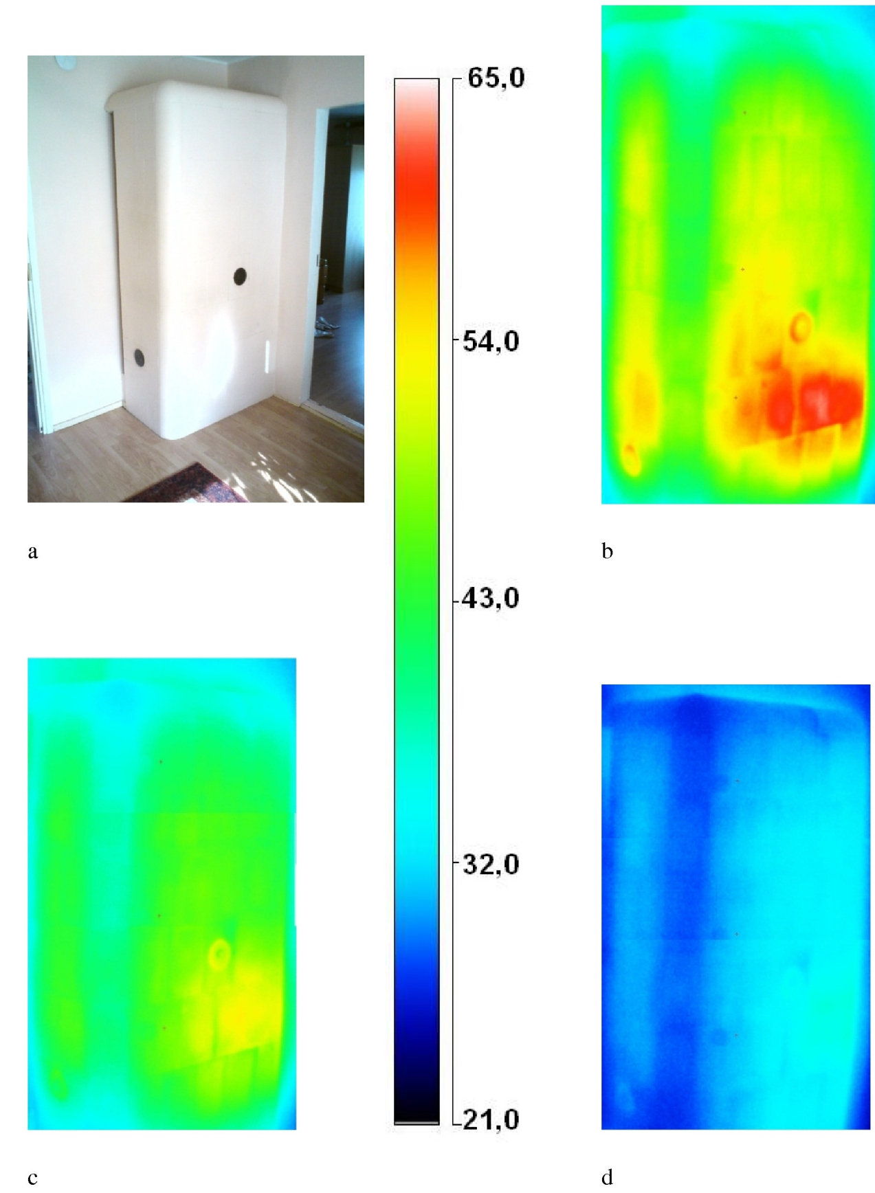
Joonis 1. Ahju termograafia a – ahju üldvaade, millest tehti termofotod; b – 4 tundi pärast sulgemist; c – 8 tundi pärast siibri sulgemist; d – 21 tundi pärast siibri sulgemist. Figure 1. Owen thermography a –the Picture of the general view of the oven; b- 4 hours after shutting down; c – 8 hours after shutting down; d- 21 hours after shutting down;
