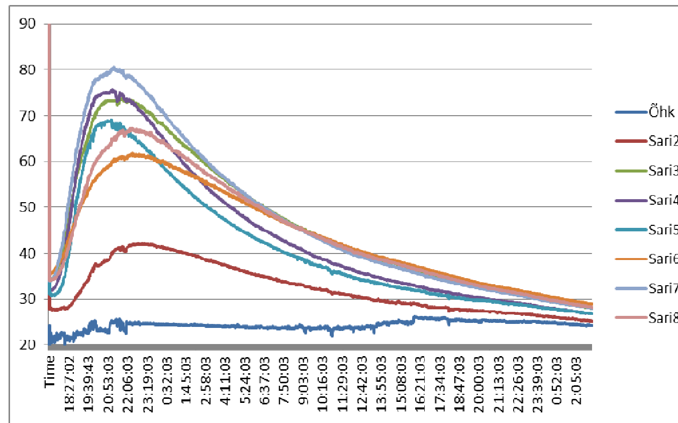
Joonis 3 Ahju pinnatemperatuuride mõõtmistulemused vaatlusperioodil Figure 3 Measurements results of surface temperatures
