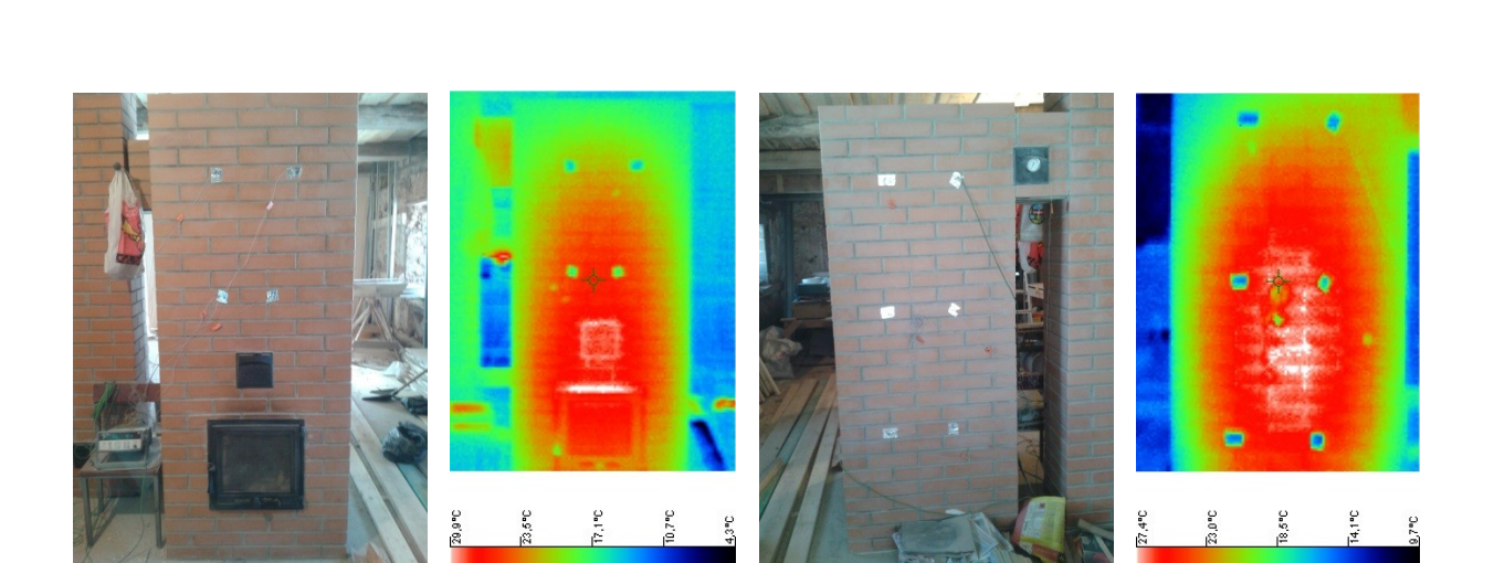
Joonis 3. Termofotod ahju eest- ja tagantvaates on tehtud 20 tundi pärast ahju kütmist
