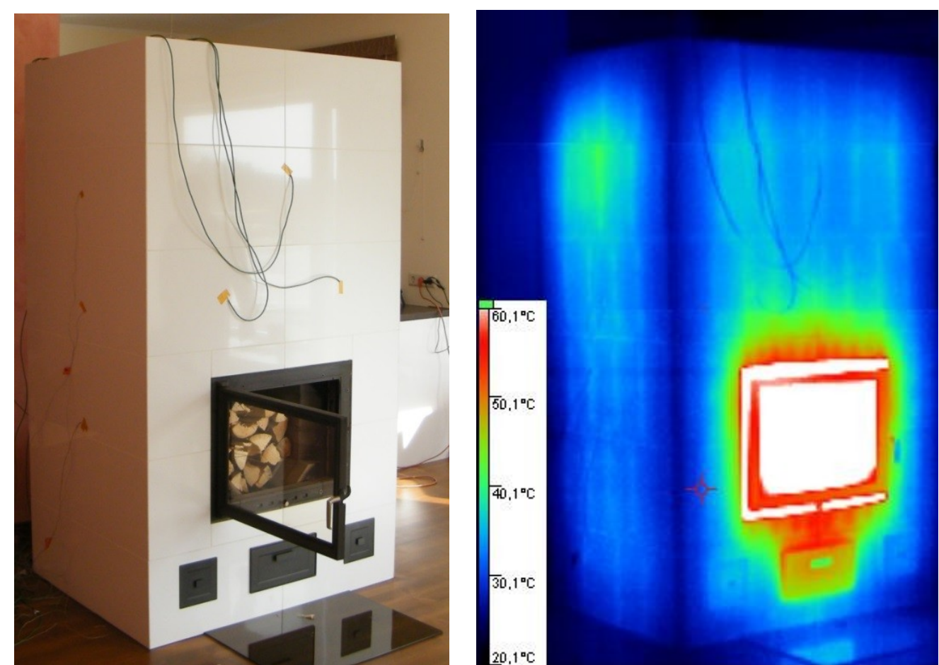
Joonis 2. Erika ahju üldvaade enne kütmist ja termopilt 4 h pärast siibri sulgemist
